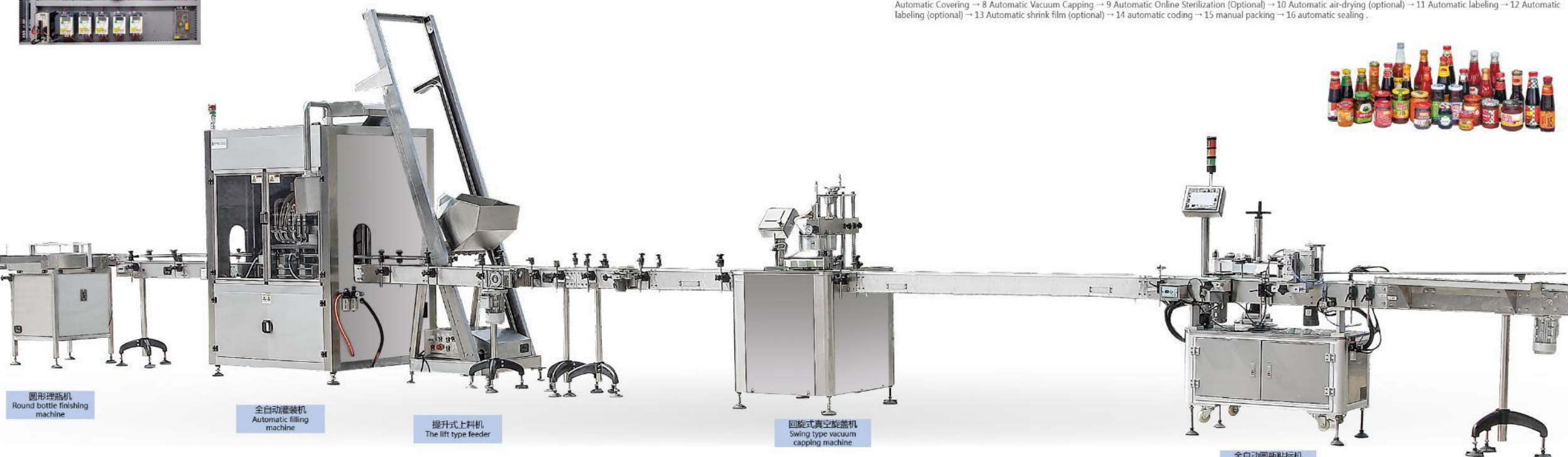
全自动圆瓶贴标机 Automatic round bottle labeling machine
